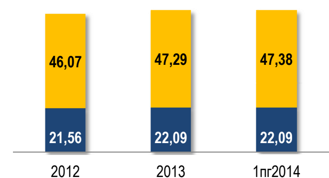
Установленная мощность подстанций, тыс. МВА
