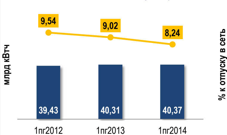
Показатели баланса электроэнергии
